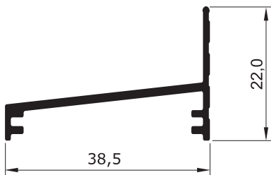
BX - 349 0,251 Kg/m
