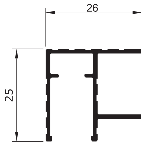
Y - 308 0,280 Kg/m
