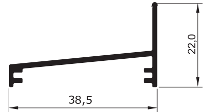
BX - 249 0,257 Kg/m
