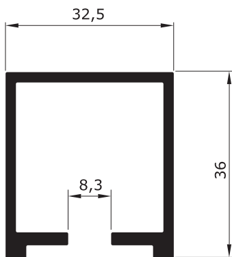
U - 164 0,708 Kg/m
