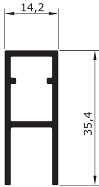
A - 022 0,420 Kg/m
