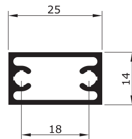
D - 082 0,349 Kg/m
