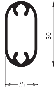
CG-087 0,359 Kg/m
