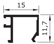
U - 482 0,115 Kg/m
