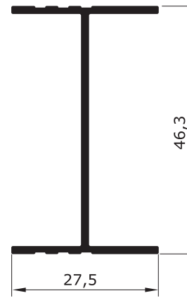
I - 155 0,389 Kg/m
