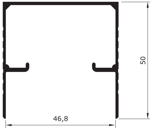
U - 655 0,645 Kg/m
