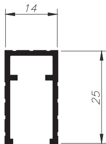
U - 652 0,255 Kg/m
