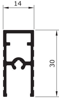
A - 087 0,366 Kg/m
