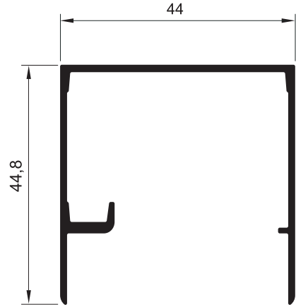
BX - 248 0,505 Kg/m
