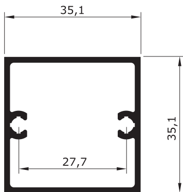
D - 081 0,643 Kg/m
