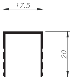
U - 654 0,170 Kg/m
