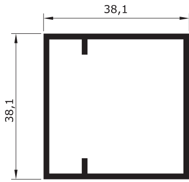
D - 102 0,627 Kg/m
