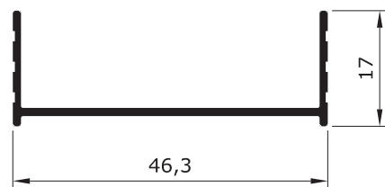
U - 653 0,246 Kg/m
