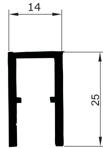
U - 396 0,285 Kg/m
