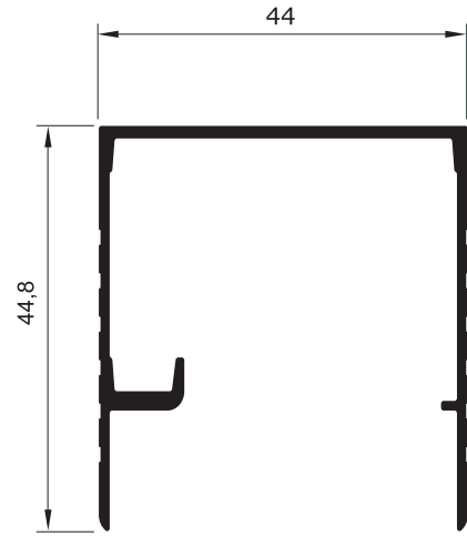
BX - 348 0,495 Kg/m
