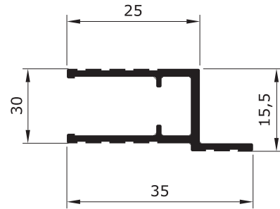
Y - 310 0,302 Kg/m
