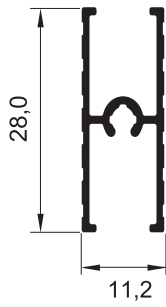
BX - 346 0,208 Kg/m
