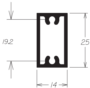
CG-021 0,329 Kg/m
