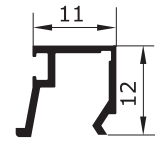
U - 522 0,100 Kg/m
