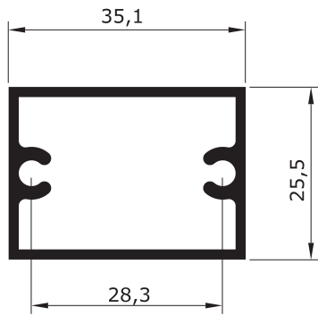
D - 055 0,580 Kg/m
