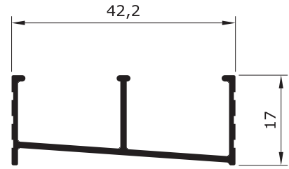
E - 256 0,256 Kg/m
