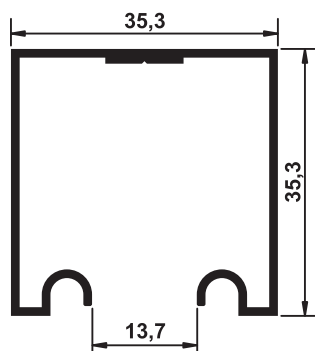
U - 1098 0,565 Kg/m
