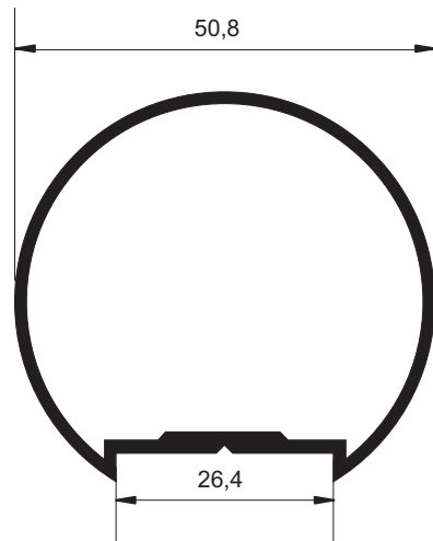
D - 094 0,650 Kg/m
