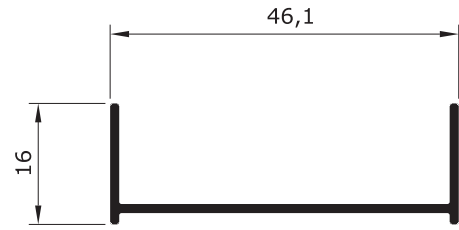
U - 399 0,245 Kg/m
