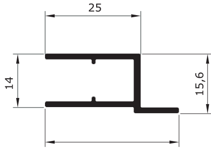
Y - 106 0,217 Kg/m
