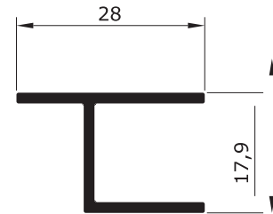
Y - 107 0,263 Kg/m
