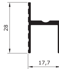
Y - 311 0,264 Kg/m
