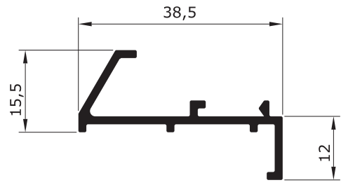
Z - 063 0,325 Kg/m
