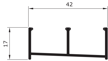
E - 117 0,334 Kg/m
