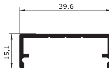
U - 496 0,338 Kg/m
