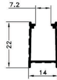
BX - 350 0,154 Kg/m
