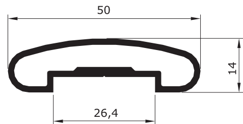
D - 095 0,544 Kg/m
