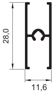
BX - 246 0,216 Kg/m
