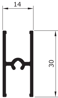
I - 083 0,321 Kg/m
