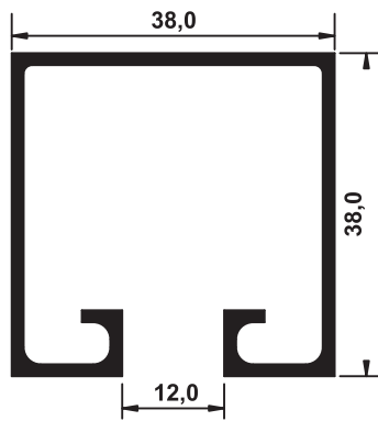
U - 990 0,740 Kg/m
