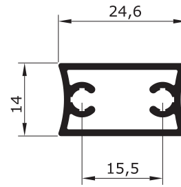
D - 056 0,343 Kg/m
