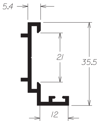
L - 519 0,297 Kg/m
