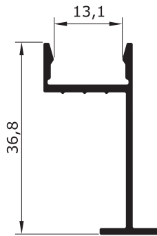
50-018 0,263 Kg/m
