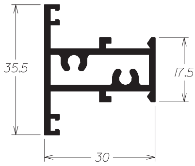
P - 075 0,590 Kg/m
