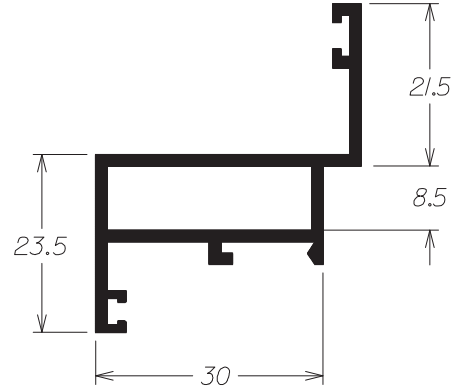
P - 121 0,533 Kg/m
