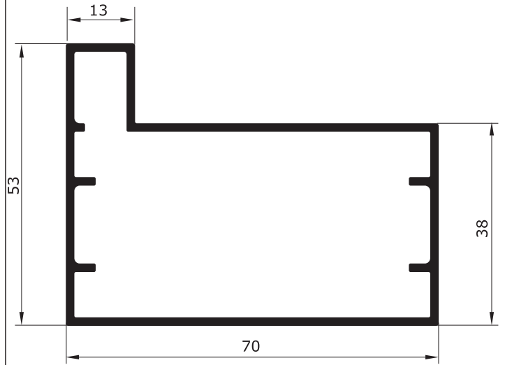
D - 141 1,111 Kg/m
