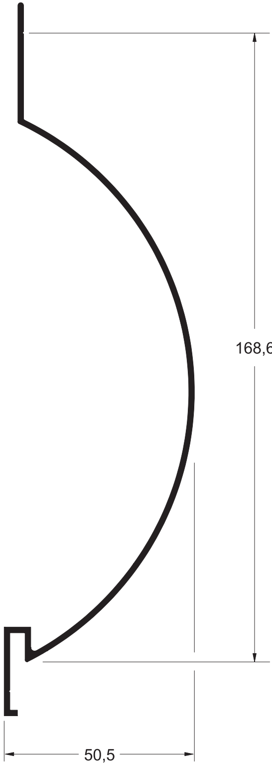
U - 1040 1,062 Kg/m
