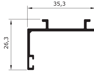
L-366 0,283 Kg/m
