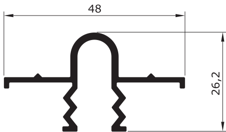
E - 364 0,458 Kg/m
