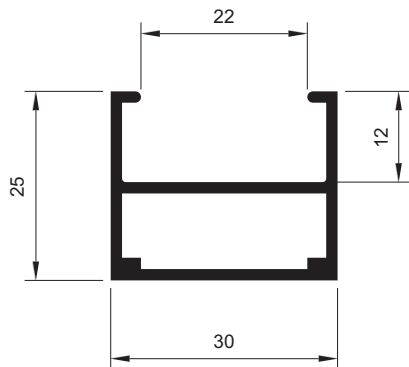
A - 209 0,463 Kg/m
