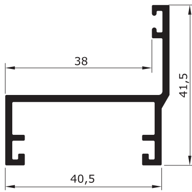
Y-181 0,570 Kg/m
