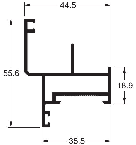
P - 272 0,775 Kg/m
