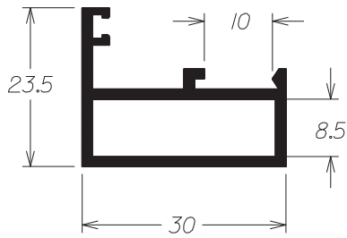
P - 064 0,408 Kg/m
