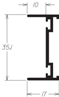
E - 150 0,295 Kg/m
