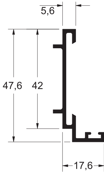
L - 521 0,368 Kg/m
