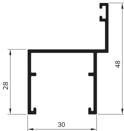
Y - 346 0,504 Kg/m
