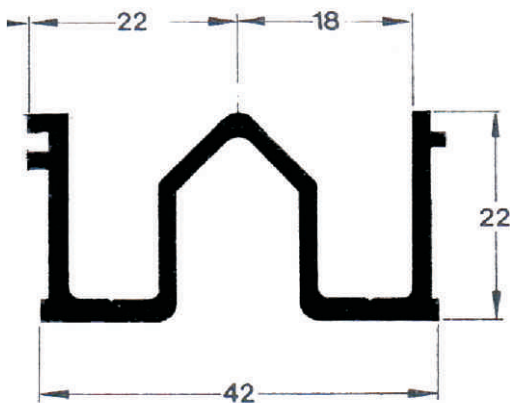
E - 487 0,600 Kg/m
