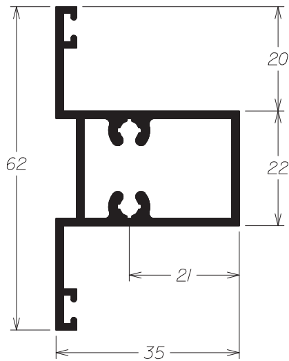
P - 419 0,726 Kg/m
