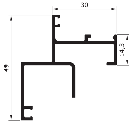
Y - 202 0,567 Kg/m
