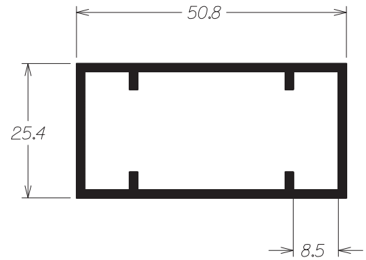
D - 079 0,650 Kg/m
