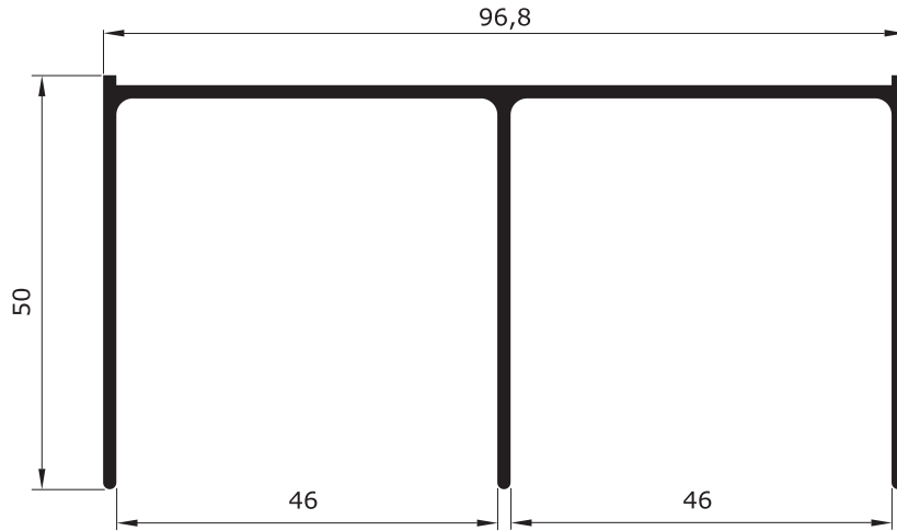
E - 363 1,043 Kg/m
