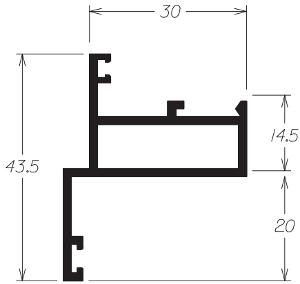
P - 120 0,533 Kg/m
