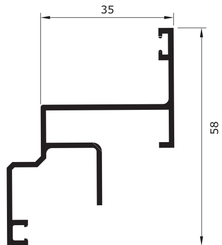
Y - 214 0,606 Kg/m
