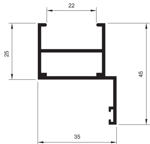
P - 575 0,583 Kg/m
