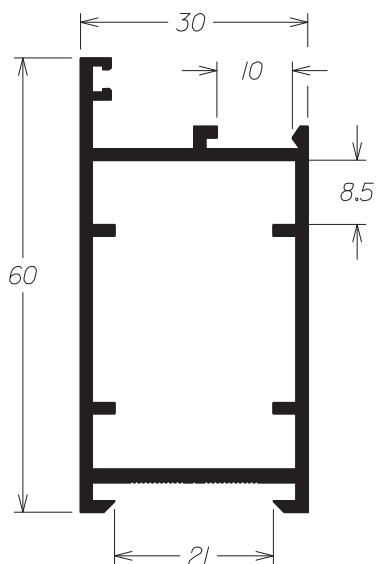
P - 270 0,780 Kg/m
