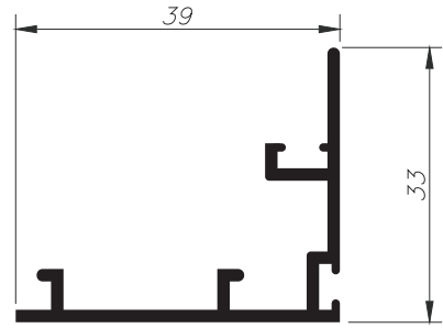
L - 517 0,402 Kg/m
