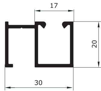
Z - 082 0,393 Kg/m
