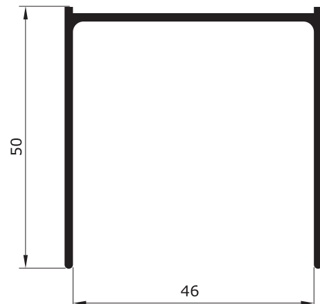
M - 027 0,636 Kg/m
