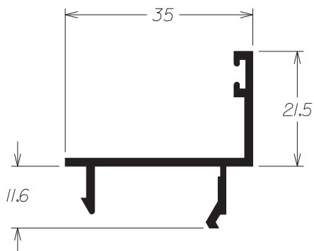
Y - 148 0,340 Kg/m
