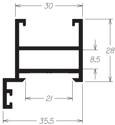
P - 273 0,615 Kg/m
