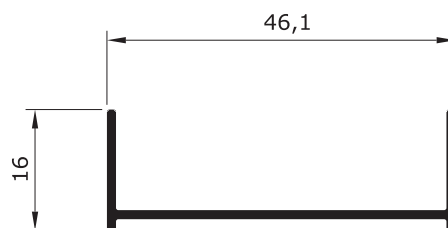
U - 399 0,245 Kg/m
