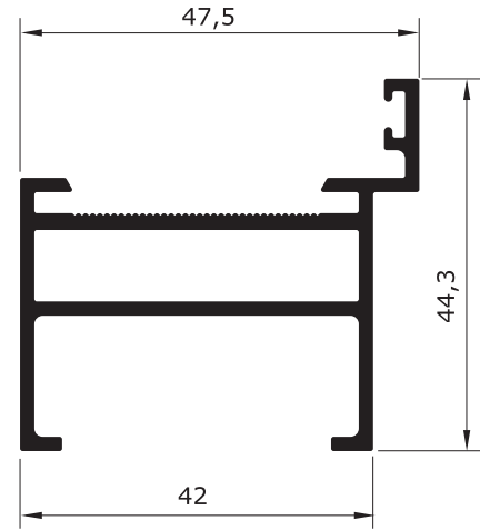
P - 280 0,855 Kg/m
