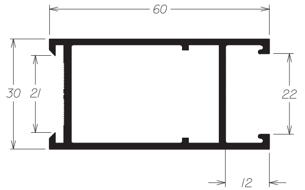
A - 144 0,829 Kg/m
