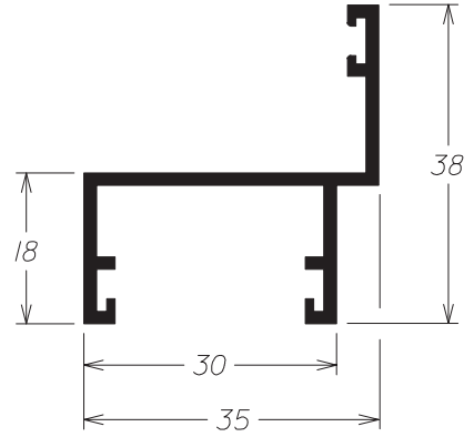
Y - 140 0,435 Kg/m
