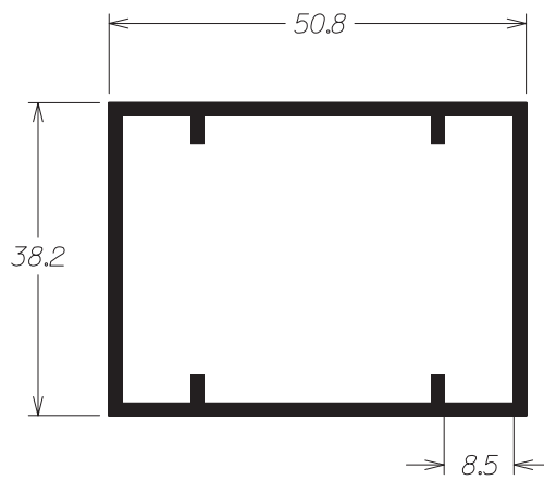
D - 078 0,755 Kg/m
