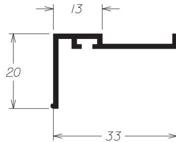
L - 387 0,210 Kg/m
