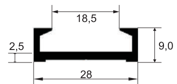
U - 690 0,260 Kg/m
