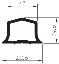
A - 213 0,254 Kg/m
