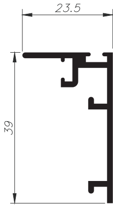
L - 518 0,366 Kg/m
