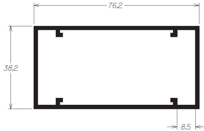
D - 069 0,945 Kg/m
